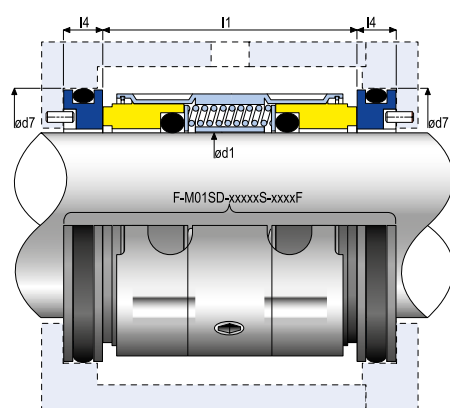
Fybroc Seal
